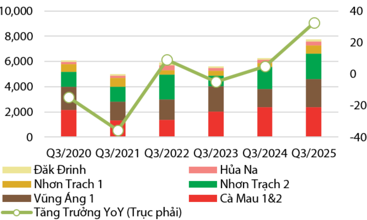
Hình 2: Doanh thu Q3 từ các nhà máy điện chính của POW (tỷ đồng)
