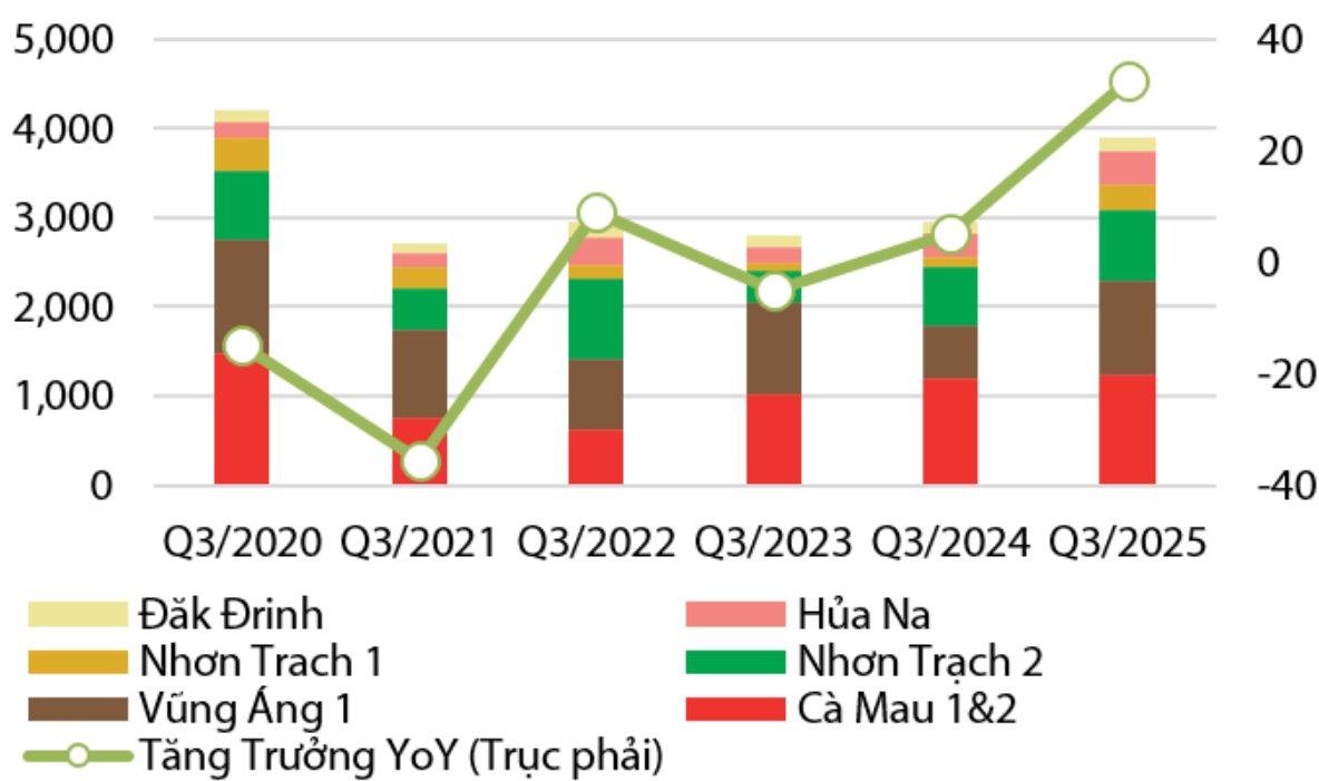
Hình 1: Sản lượng điện phát Q3 từ các nhà máy chính của POW (triệu kWh) và mức tăng trưởng YoY (%)
